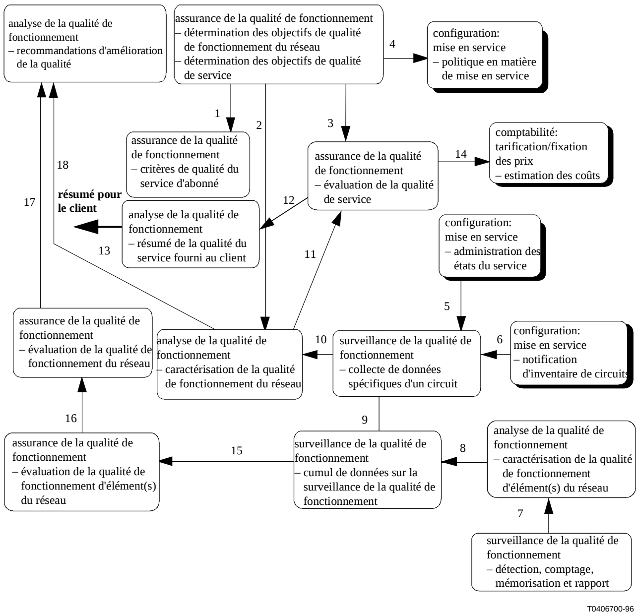
Figure I.11/M.3400 – Assurance de la qualité de fonctionnement
