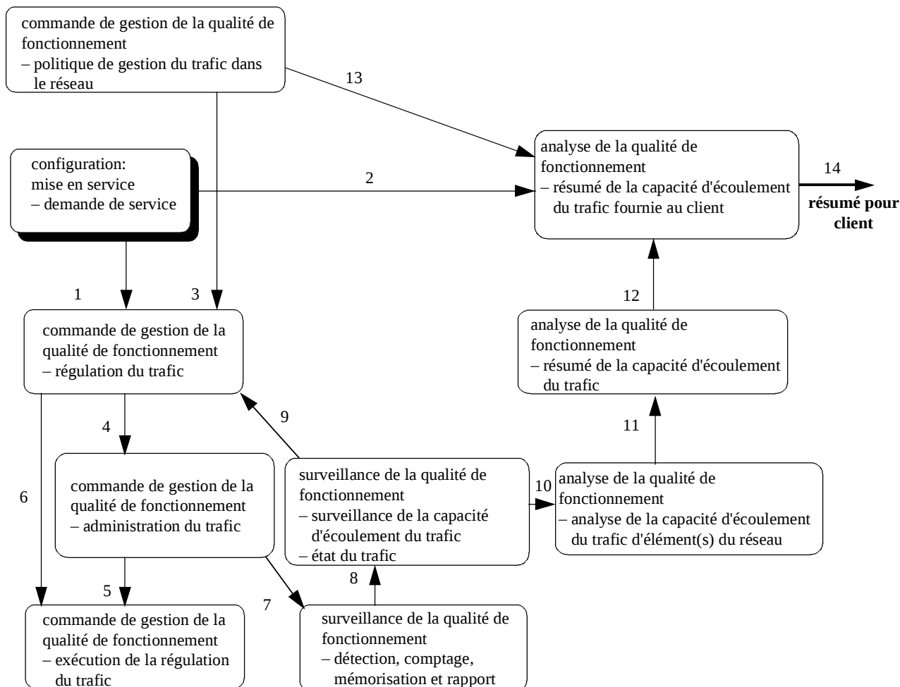
Figure I.15/M.3400 – Régulation du trafic associée à la clientèle
