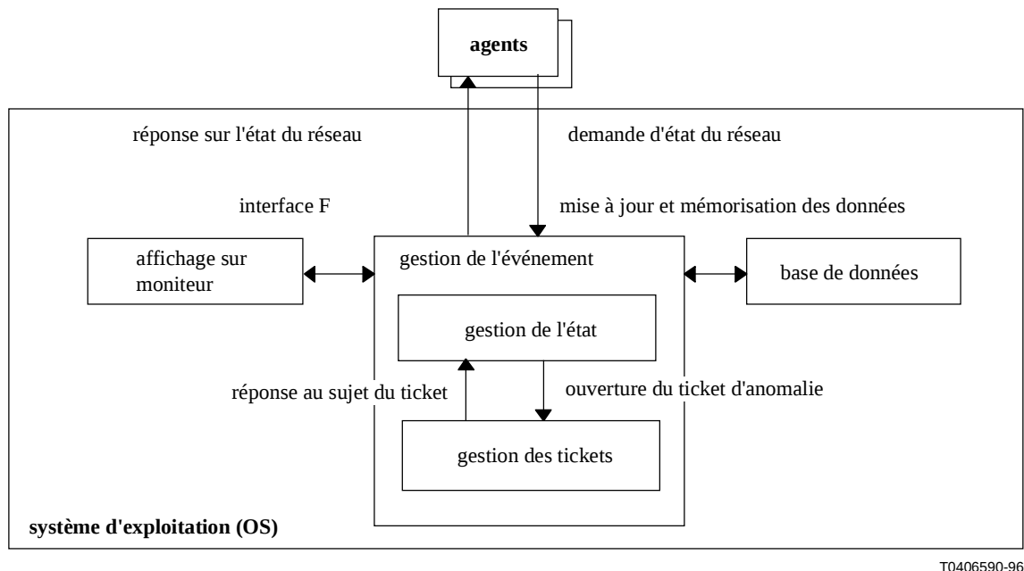
Figure 4/M.3400 – Localisation des dérangements dans le réseau
